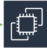
virtuális gép
