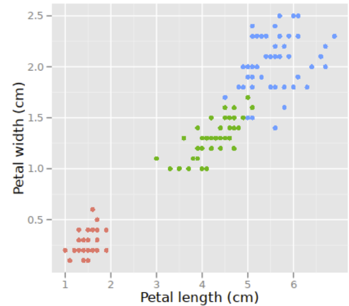
Iris adathalmaz
